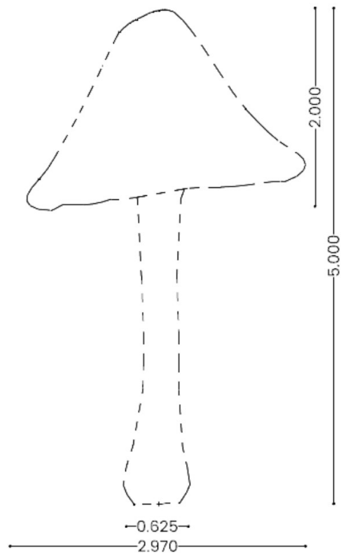
Figuur 1 – Aanzicht van het object met maatvoering
